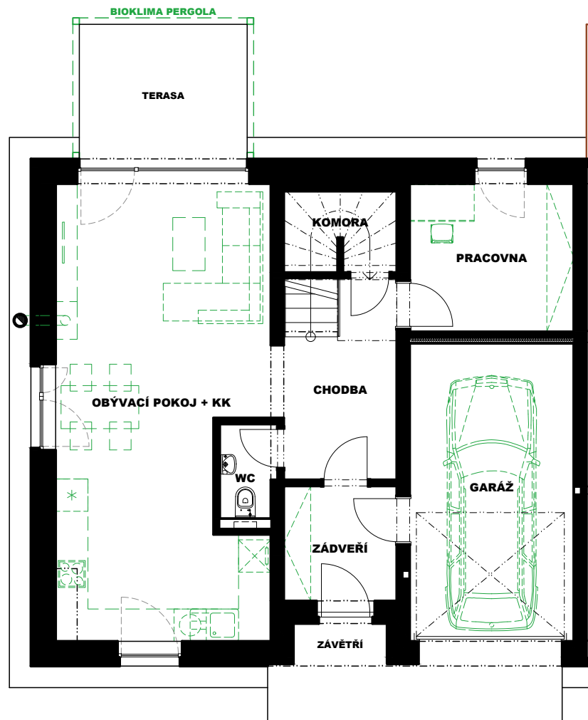
PŮDORYS 1.NP
